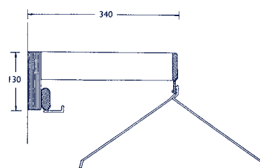
DLM 1100-KH KH avec cintres et crochets tournés vers l'extérieur
