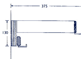
DLM 1100-HH avec 2 rangées de crochets, dont celle à l'avant tournée vers l'intérieur ou l'extérieur
